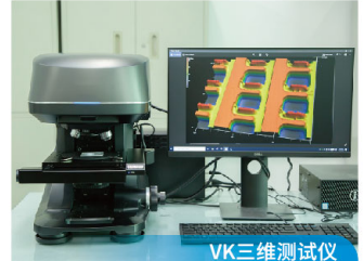
VK三维测试仪
